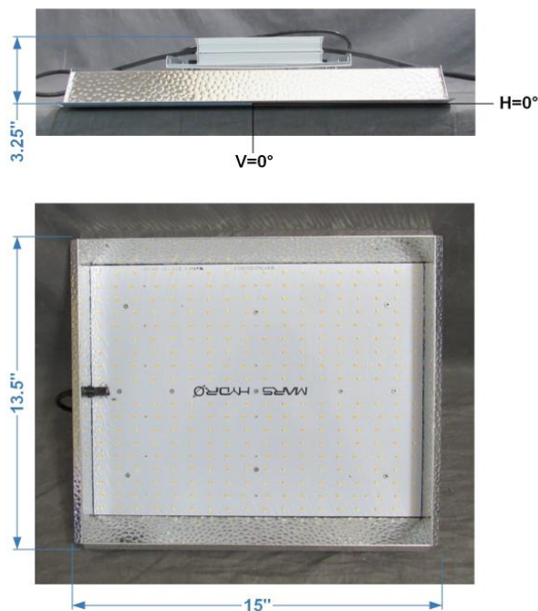
FIG. 1 LUMINAIRE
